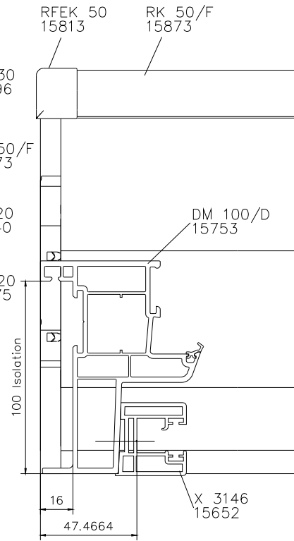
Coupe horizontale
