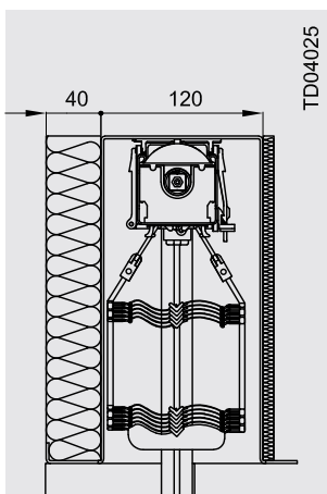
MODULO crépissable avec isolation arrière 40 mm (également possible sur système visible)
