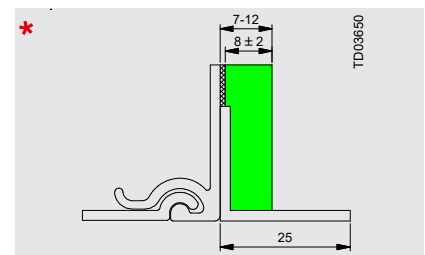
Plaque en Styrodur 8 mm et cornière 25 mm (option 2)
