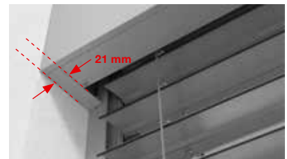
Frise bilatérale (standard sur INTEGO)
