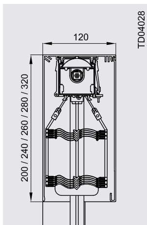
MODULO avec capot visible (extrudé)
