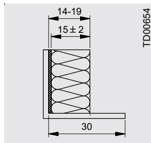
Plaque en Styrodur 15 mm
