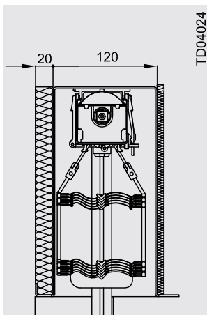
MODULO crépissable avec isolation arrière 20 mm (également possible sur système visible)
