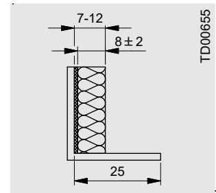
Plaque en Styrodur 8 mm
