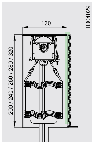
MODULO crépissable (capot en tôle pliée)
