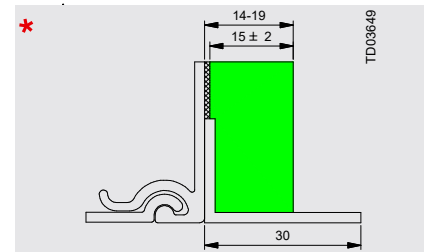
Plaque en Styrodur 15 mm et cornière 30 mm (option 1)
