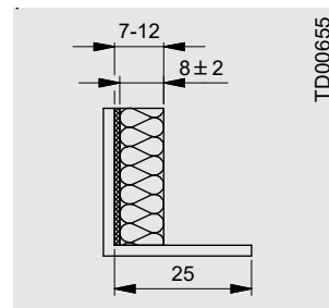
Plaque en Styrodur 8 mm
