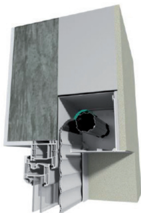
ITE En neuf ou rénovation, dans le doublage de l'isolation
