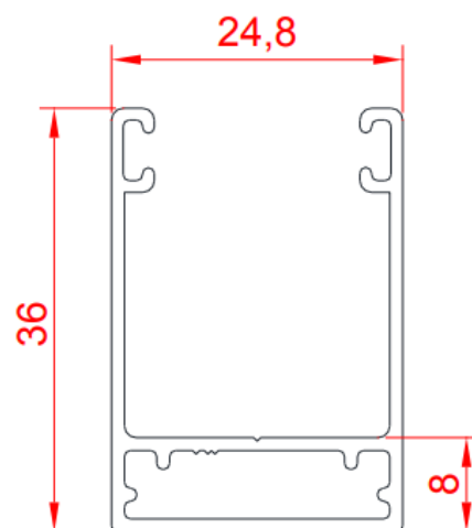
Illustration des coulisses réduites de l'Allegro Tradi
