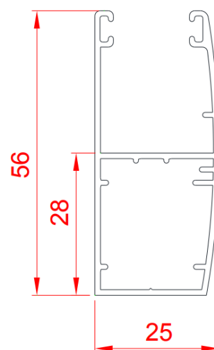
Illustration des coulisses de l'Allegro Tableau
