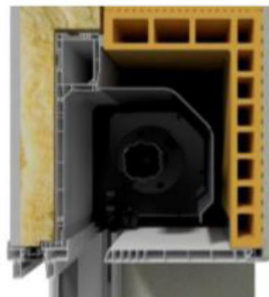
Représentation avec sous-face linteau 215
