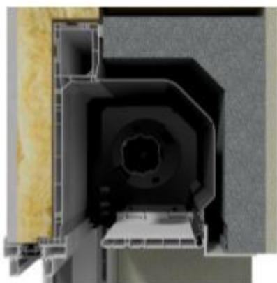
Représentation avec cornière 40x60
