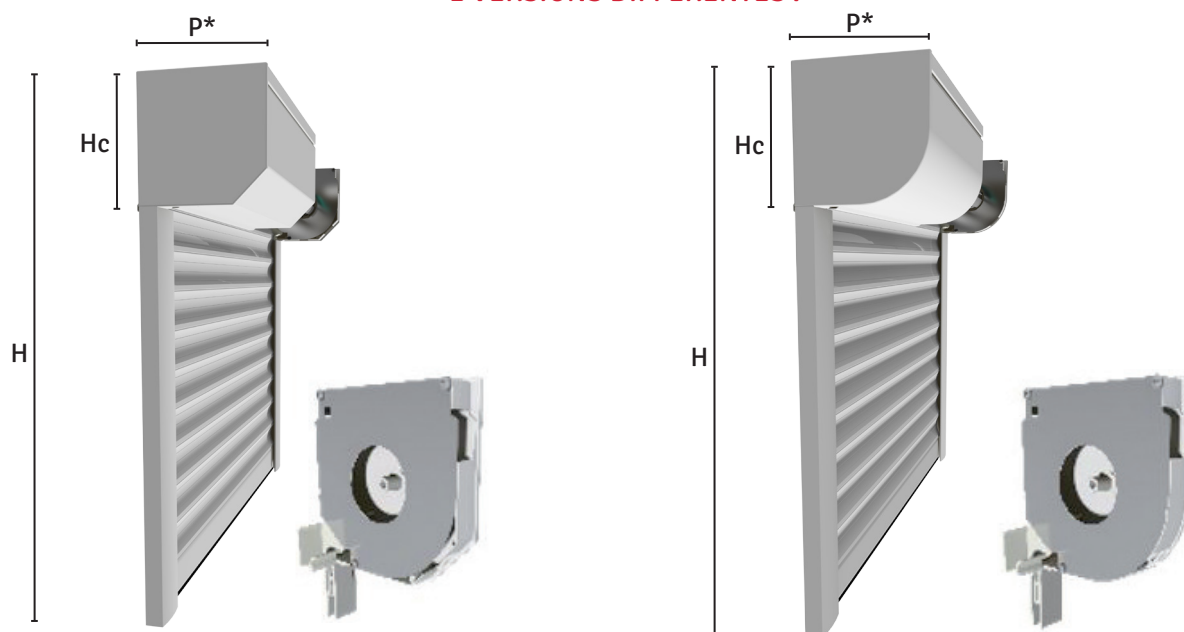
Coffre Pan Coupé avec jous aluminium : pour une meilleure finition
