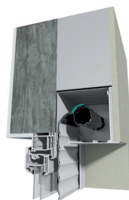
ITE En neuf ou rénovation, dans le doublage de l'isolation
