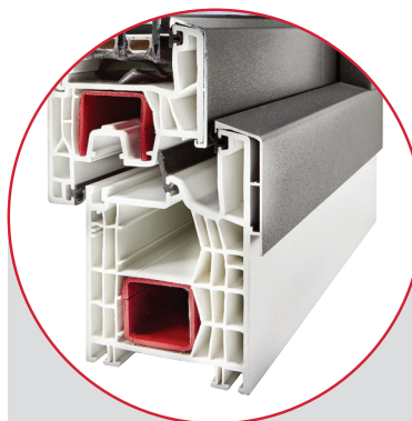
Modèle AluClip capotage court
