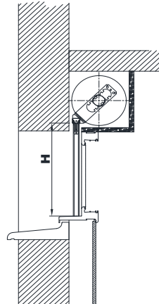
Pose en coffre menuisé
