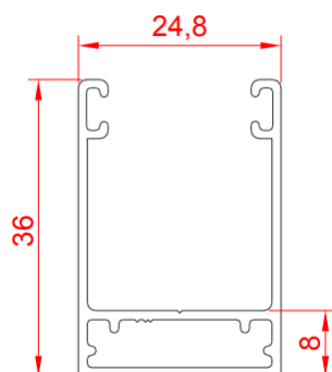
Coulisse réduite de l'Allegro Tradi
