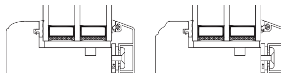
Profil Quart Ellipse
