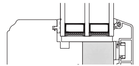
Profil Quart Doucine
