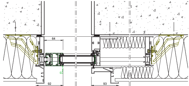
COUPE HORIZONTALE
