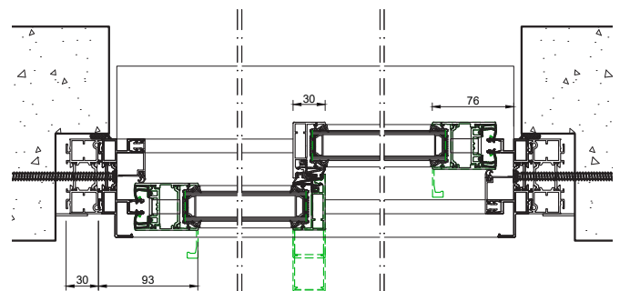
COUPE HORIZONTALE
