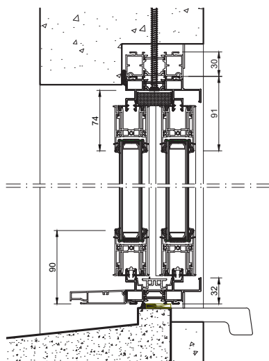
COUPE VERTICALE
