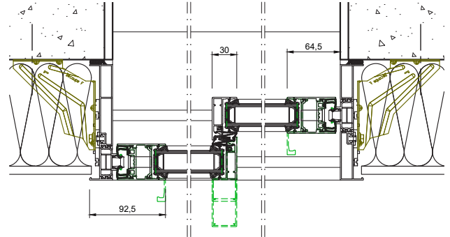
COUPE HORIZONTALE
