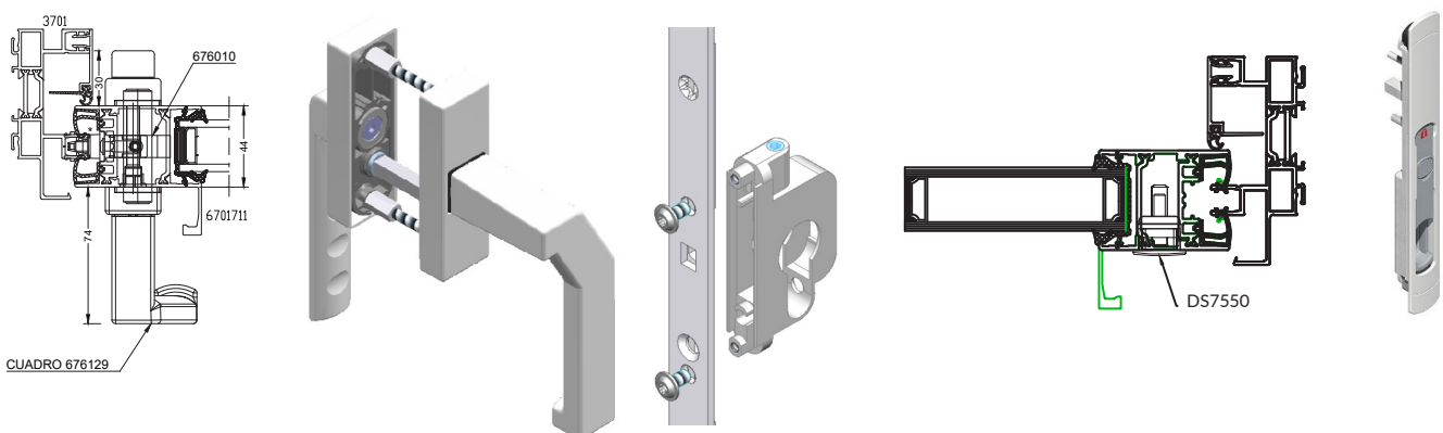
Ensemble intérieur - extérieur (côté extérieur saillie réduite)
