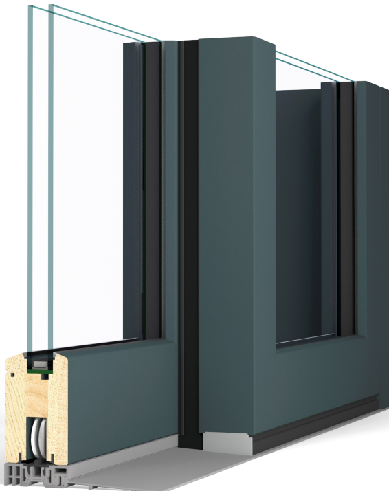
Coulissant levant seuil rénovation sur dalle existante Couleur : gris granite - RAL 7026 Profil intérieur : Pente Profil extérieur : Pente
