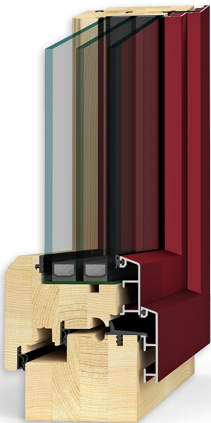
UNI 9 Couleur : intérieur : incolore mat, extérieur : rouge vin - RAL 3005 Profil intérieur : Doucine
