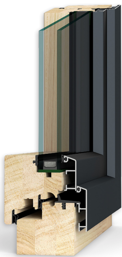
UNI 8 Couleur : intérieur : incolore mat, extérieur : gris anthracite - RAL 7016 Profil intérieur : Carré
