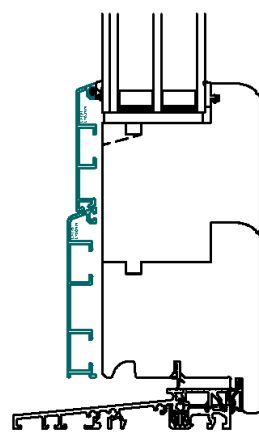
Seuil aluminium 110 mm
