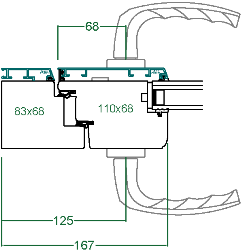
Ensemble int./ext. béquilles Atlanta
