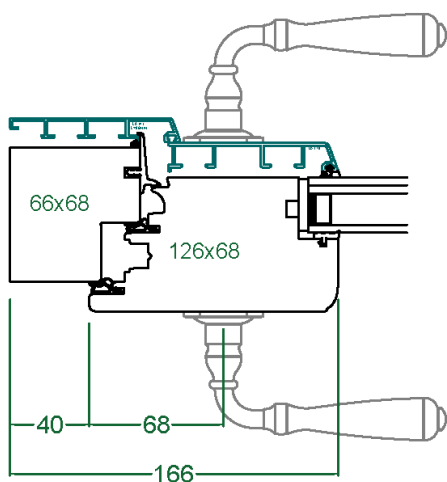
Ensemble int./ext. béquilles Entraygues
