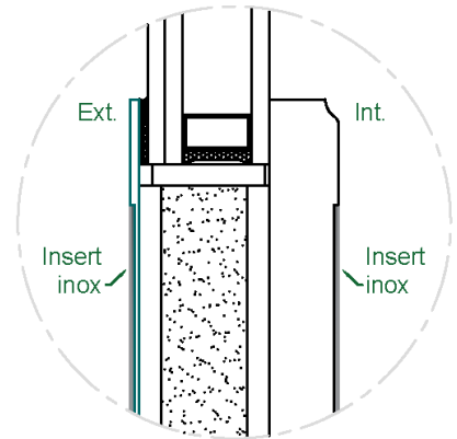
Avec insert inox intérieur
