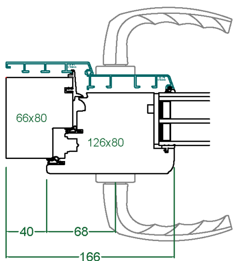
Ensemble int./ext. béquilles Atlanta
