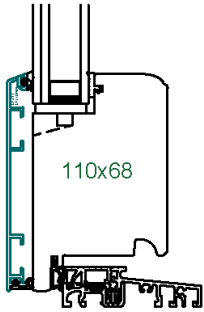
Seuil aluminium 70 mm
