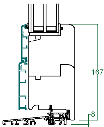
Seuil aluminium 110 mm
