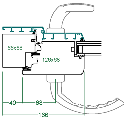
Elément de tirage ext. Bouton Stuttgart Béquille int. Stuttgart
