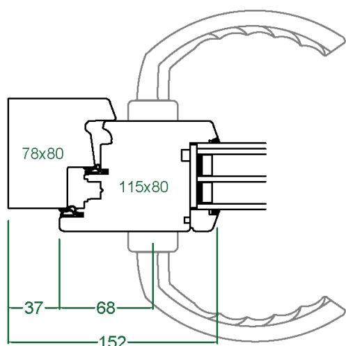
Ensemble int./ext. béquilles Stuttgart
