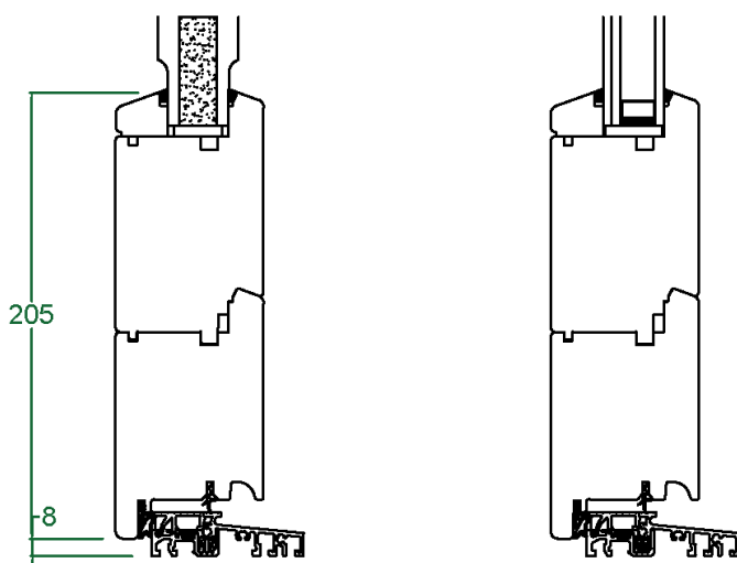
Seuil aluminium 70 mm
