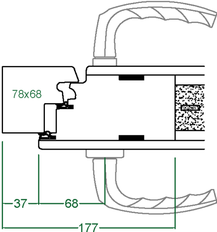
Ensemble int./ext. béquilles Atlanta
