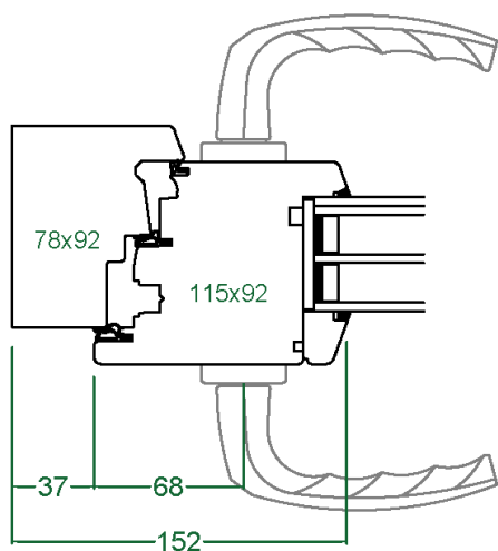
Ensemble int./ext. béquilles Atlanta
