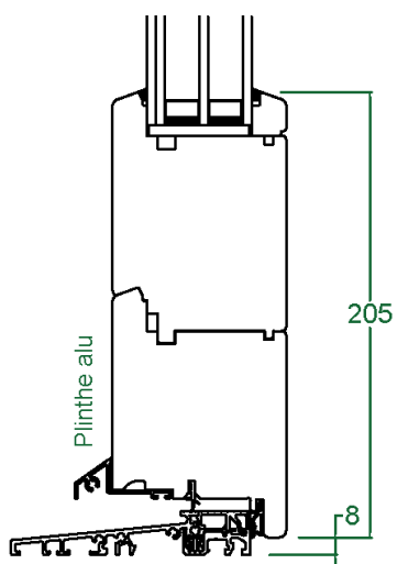
Seuil aluminium 110 mm
