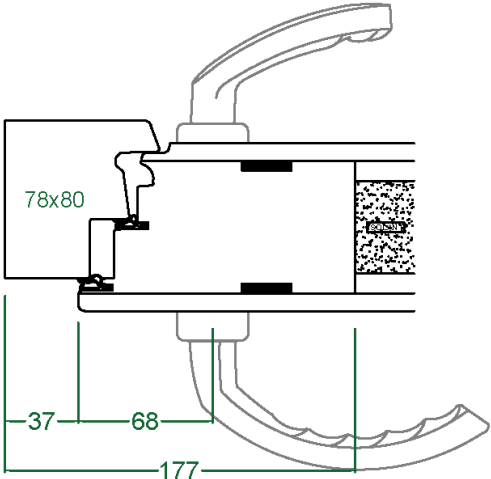
Elément de tirage ext. Fer à cheval Stuttgart Béquille int. Stuttgart
