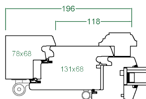
Déduction cotes pour dimensions grilles
