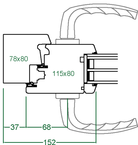
Ensemble int./ext. béquilles Atlanta
