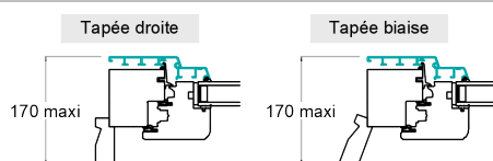
Petits bois collés sans intercalaire fictif
