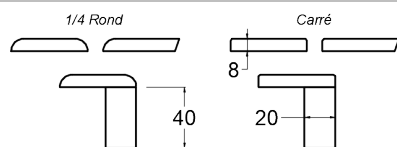
Petits bois collés
