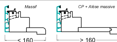
Petits bois collés - Incliné
