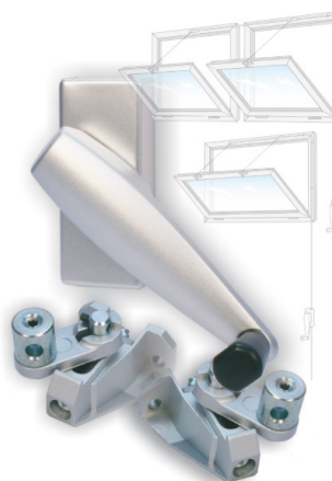
Manoeuvre ferme imposte par biellette type MAGISTRAL
