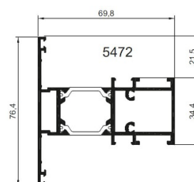
MENEAU
