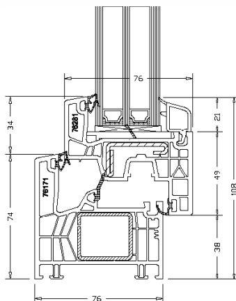
Battement recouvrement
