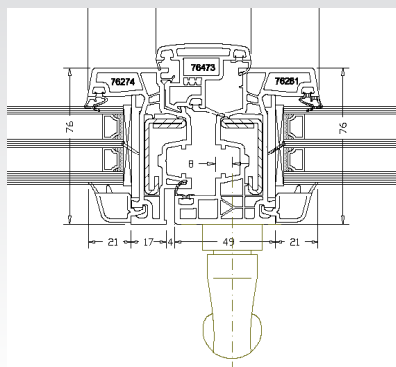
Battement recouvrement
