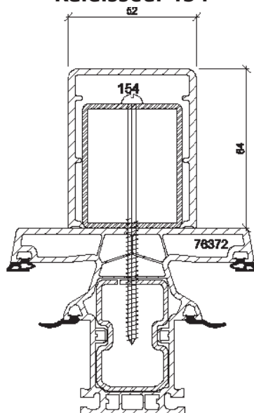
Raidisseur 154
